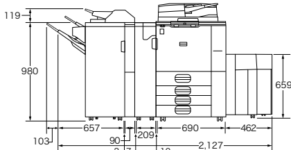
3000枚フィニッシャー SR4150 インサートフィーダー CI4040 紙折りユニット FD4010 A4大量給紙トレイ RT4080 imago トレイサイズ拡張キット タイプ36 装着時
