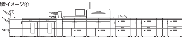
RICOH Pro C9500 3500枚フィニッシャー SR5120 5000枚スタッカー SK5040 2台 インサートフィーダー CI5040
