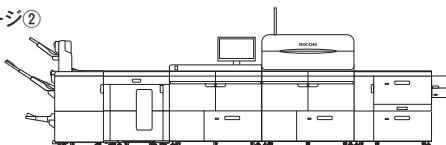
RICOH Pro C9500 3500枚フィニッシャー SR5120 5000枚スタッカー SK5040 エアピック式A3LCT RT5150 A3LCT 長尺用紙拡張キット タイプS9 SR5000シリーズ用 長尺紙排トレイ タイプS6
