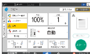
コピー画面
