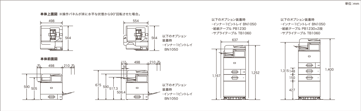
RICOH IM C431 の外形寸法
