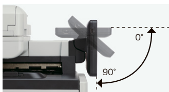
※写真は、RICOH IM C431Fの場合。 RICOH IM C431Fの場合は、20°～90度。
