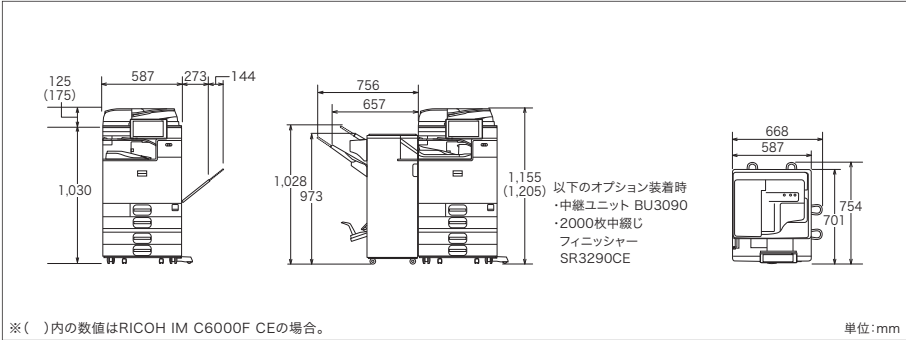
RICOH IM C6000F CE/C4500F CEの外形寸法
