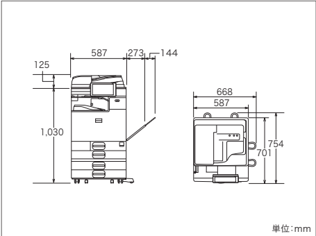
RICOH IM C3000F CE/C2500F CEの外形寸法
